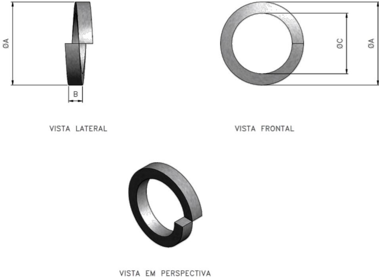
Figura 1 - Vistas da Arruela de Pressão
